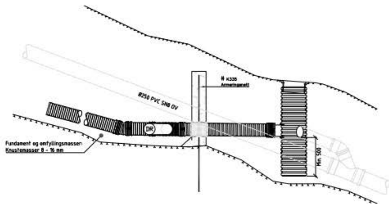
SNITT A-A Drensledning m/ sandfang 1:20
