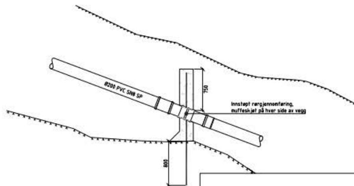
SNITT B-B 1:20
