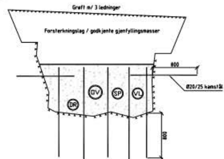
SNITT C-C 1:20
